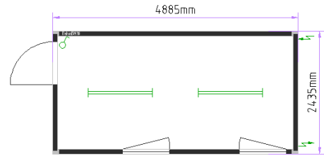
16-и футовый офисный контейнер
