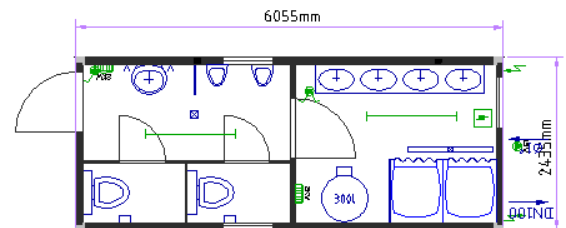
20-и футовый сантехнический блок-контейнер
