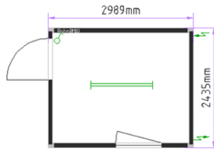
10-и футовый блок-контейнер
